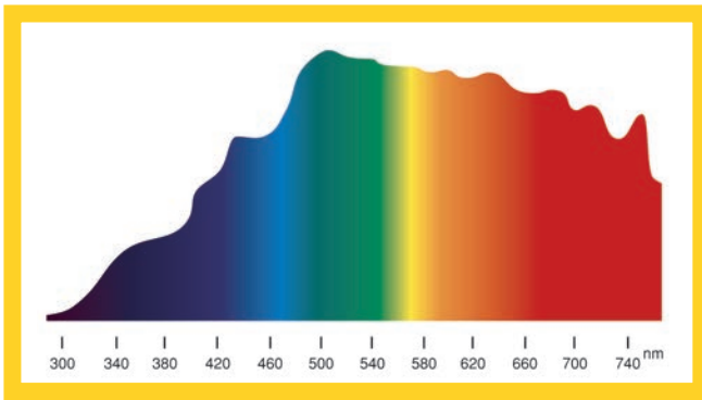
Spektrale Zusammensetzung des natürlichen Tageslichts
